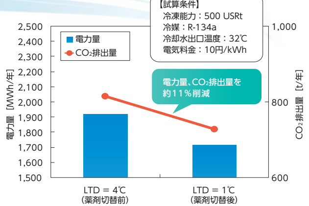
◆オルブレイドJシリーズへの切替えによる電力量・CO 2 排出量削減の試算例
